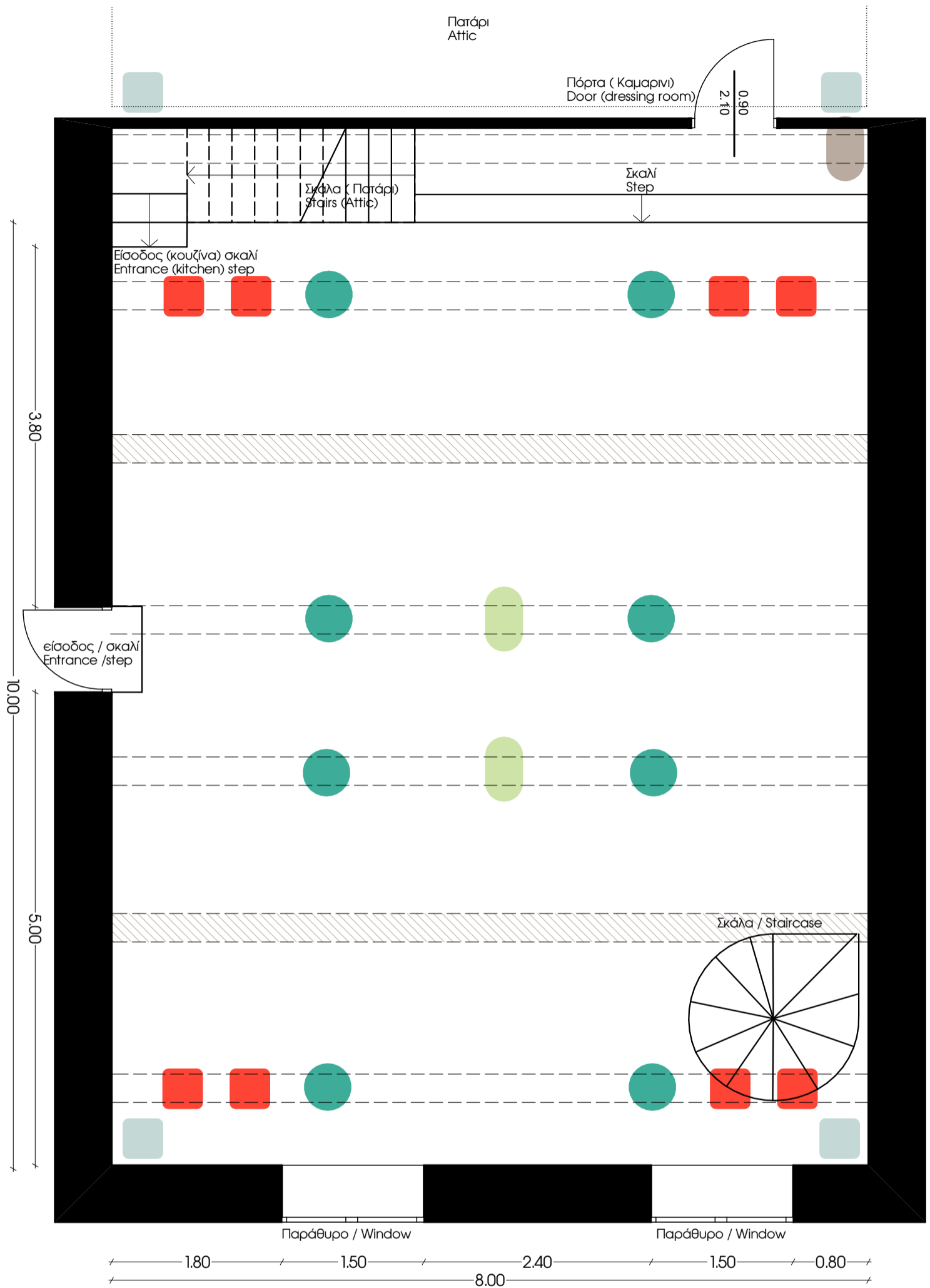
ΚΑΤΟΨΗ / κλίμακα 1:50 PLAN / scale 1:50
